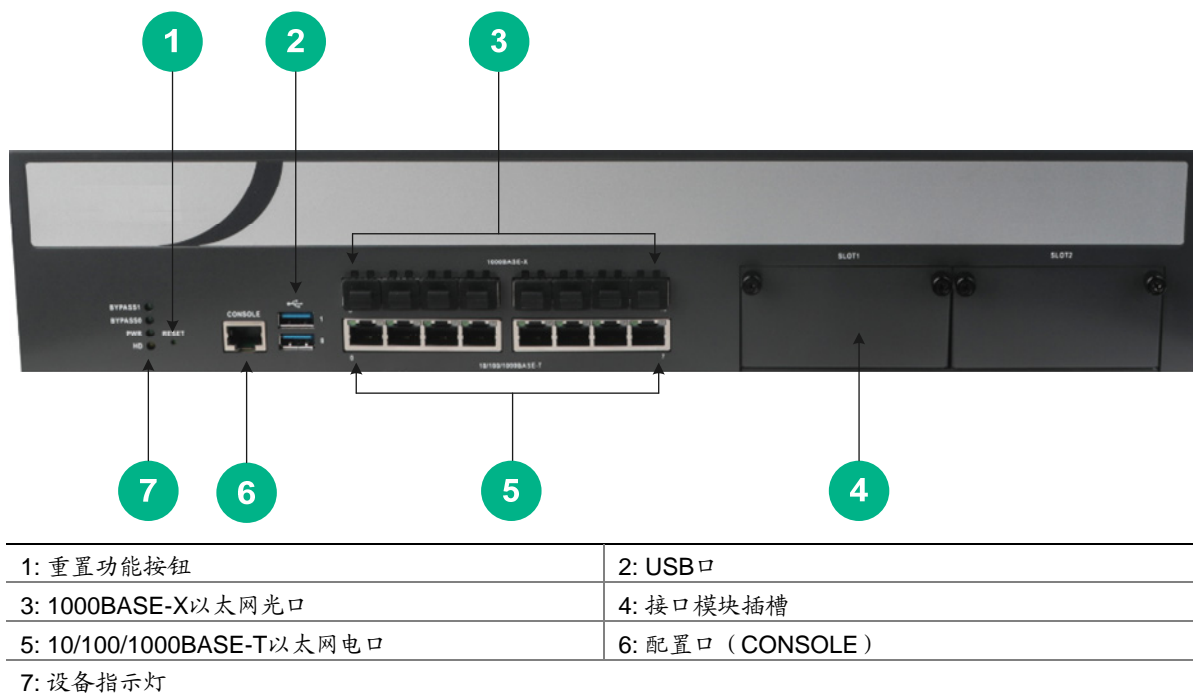
图A-2 UNIS XScan-G20 设备前视图
