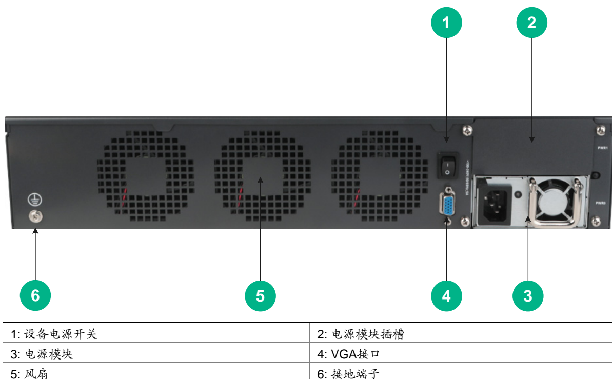
图A-4 UNIS XScan-G20 设备后视图
