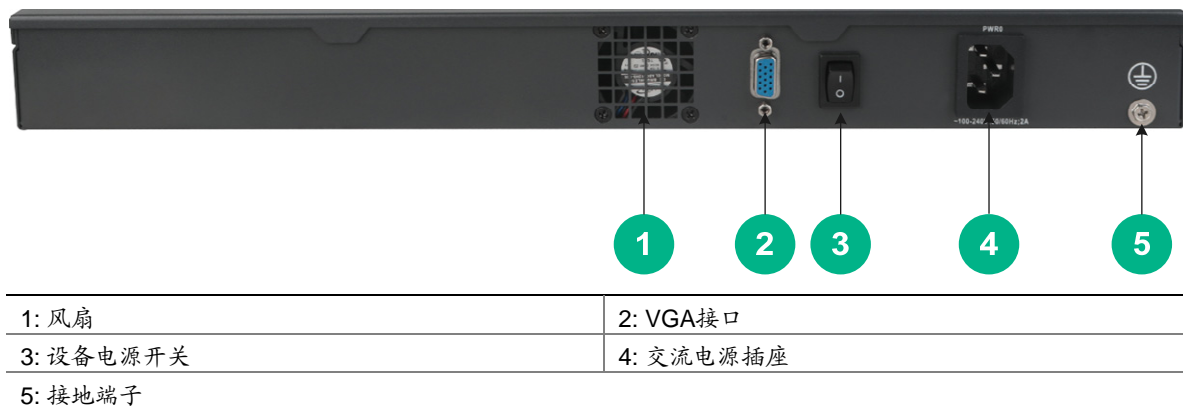
图A-3 UNIS XScan-G10 设备后视图
