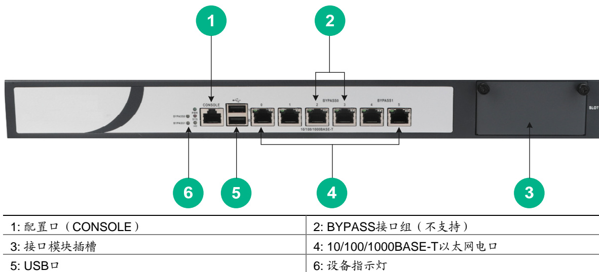
图A-1 UNIS XScan-G10 设备前视图
