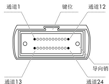
图1-3 24 芯光纤的 MPO 连接器俯视图
