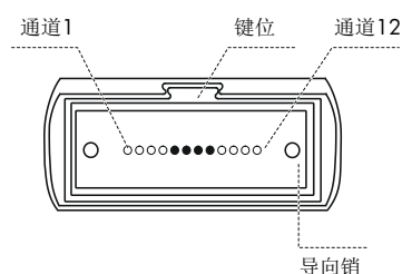
图1-2 12 芯光纤的 MPO 连接器俯视图
