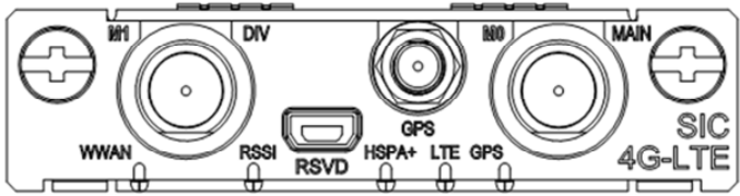
图1-4 SIC-4G-LTE-M 模块面板
