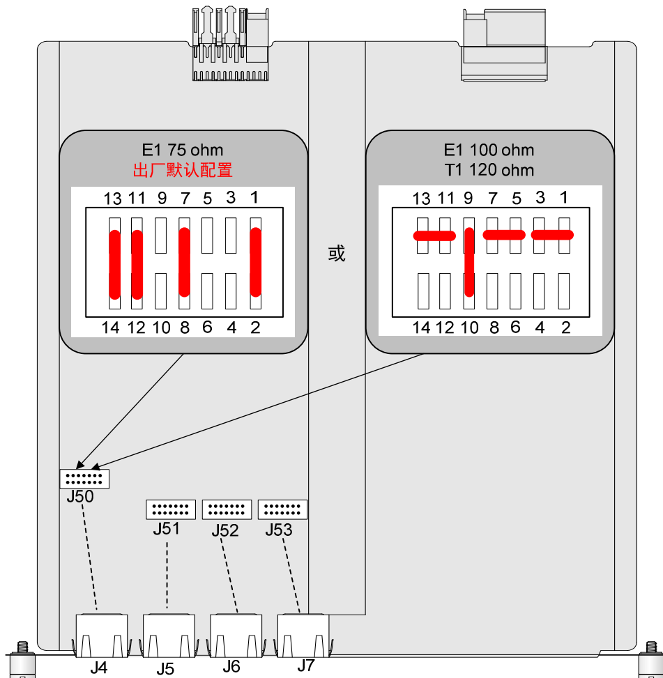
图2-7 HMIM-4E1T1 接口跳线说明
